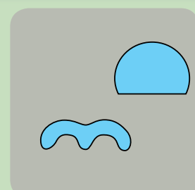
Bukan segi banyak
