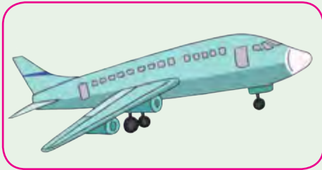
Deru pesawat merupakan contoh resonansi yang merugikan.
