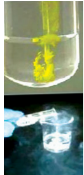
Sumber : Dok. Kemdikbud Gambar 5. 7 Pembentukan endapan Timbal Iodida
