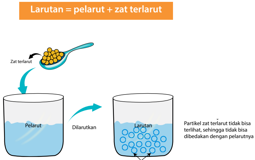
Sumber: Dok. Kemdikbud Gambar 2.20 Pelarut, zat terlarut, dan larutan
